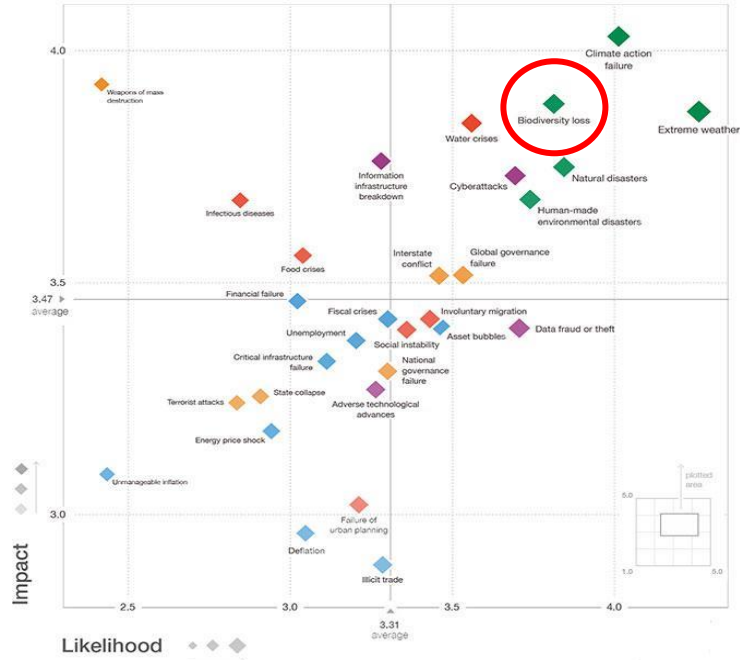
> ABB. 2 Übersicht der globalen Grenzen und deren Zustand (links, Quelle: Rockström et al., 2009) und Übersicht der grössten Risiken für die Gesellschaft und die Wirtschaft je nach Auswirkungen und Wahrscheinlichkeit mit der Biodiversität, die rot umrandet ist (rechts, Quelle: WEF; Global Risks Report 2021).
